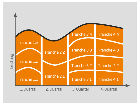
Abb. 2: Aufteilung eines Fahrplans in vertikale Tranchen
